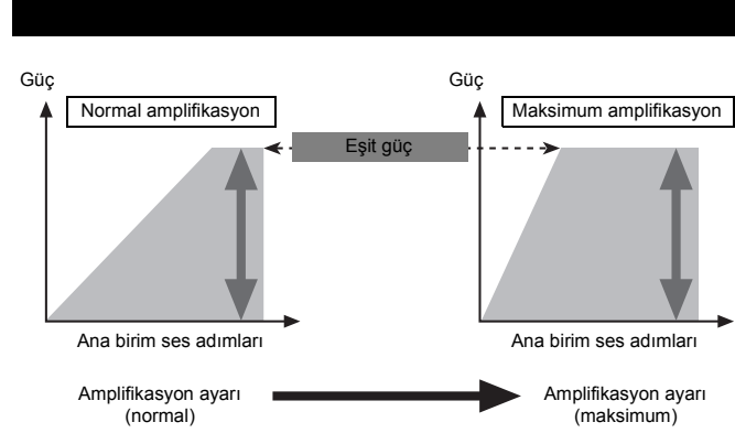
Şekil 2 Ana birimin amplifikasyon ayarı ve çıkış gücü arasındaki ilişki
