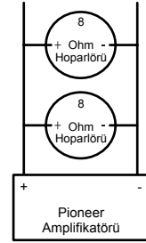
A & B Kanalları 4 Ohm'luk Kurulum
