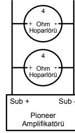
Alt Kanal 2 Ohm'luk Kurulum
