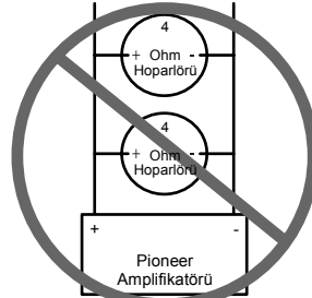
A & B Kanalları 2 Ohm'luk Kurulum
