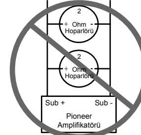
Alt Kanal 1 Ohm'luk Kurulum
