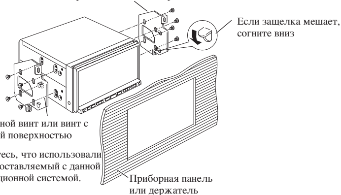
Заводской радио-монтажный кронштейн
